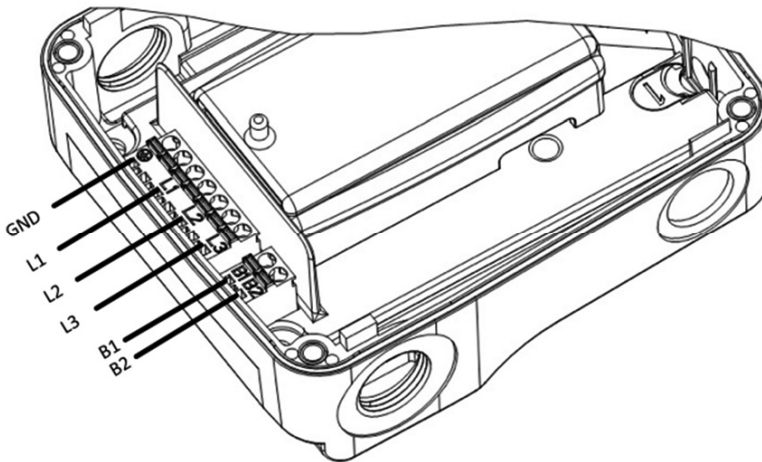
Abbildung 3: Elektroschema.
